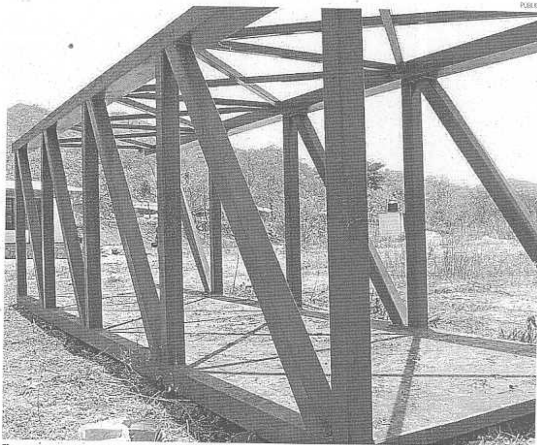
El nuevo puente ya está listo para ser instalado y fue financiado con recursos del Fonden
